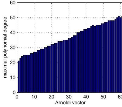
(d) polynomial degree of Arnoldi vectors
